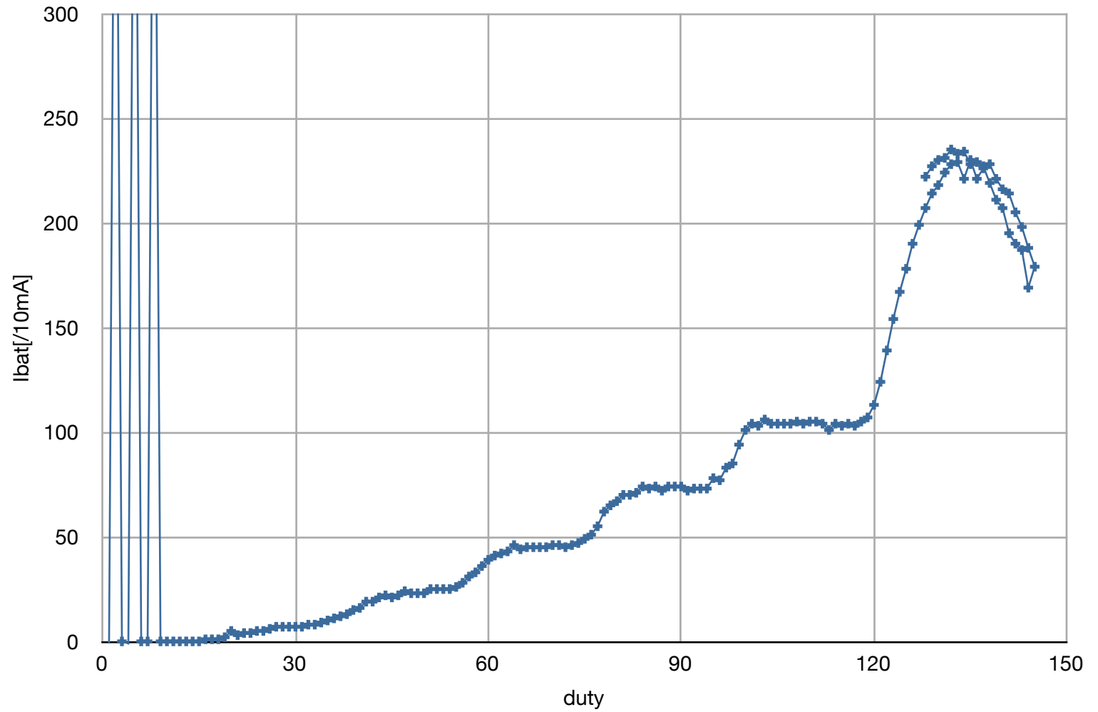
SB-1.5V500MA 100KHz
