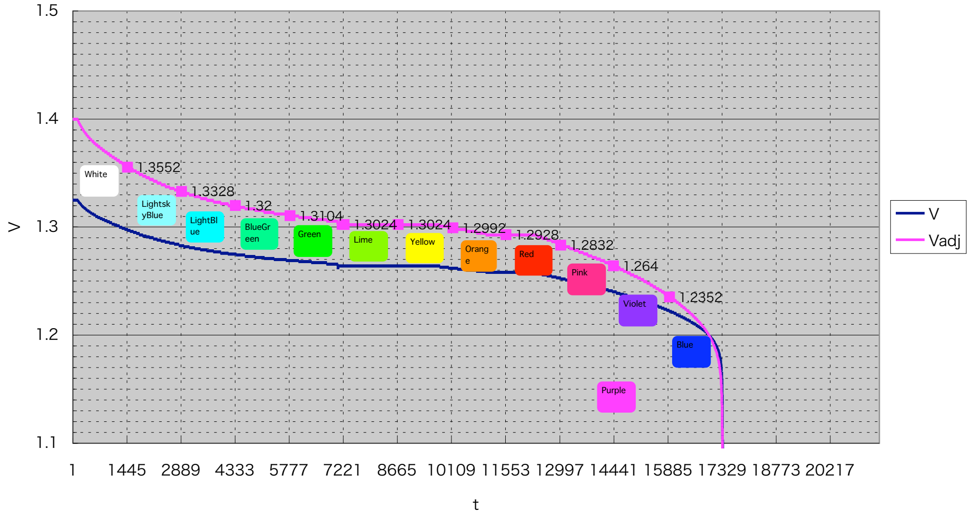
放電特性NiMH/GP2400mAh 0.5.4表示色B
