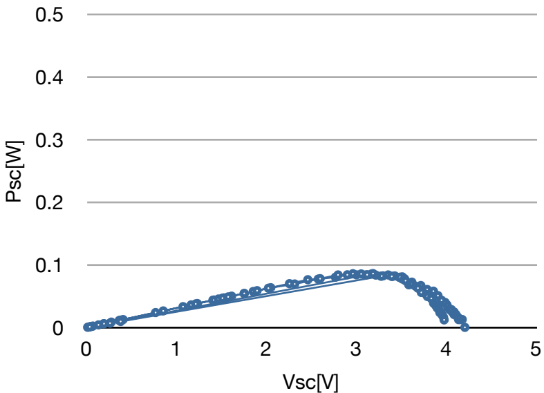
電力・電圧
