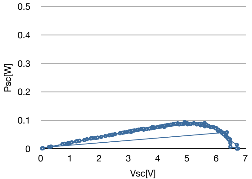
電力・電圧
