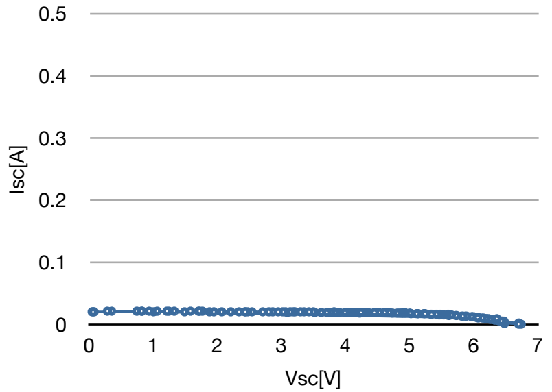
電流・電圧
